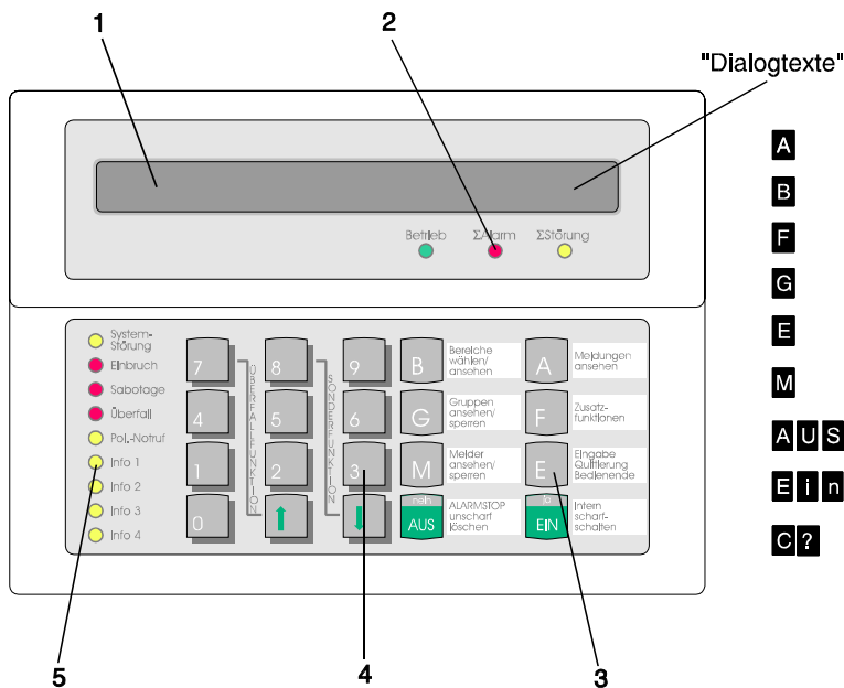
Abb. Bedienteil 012540/012541
